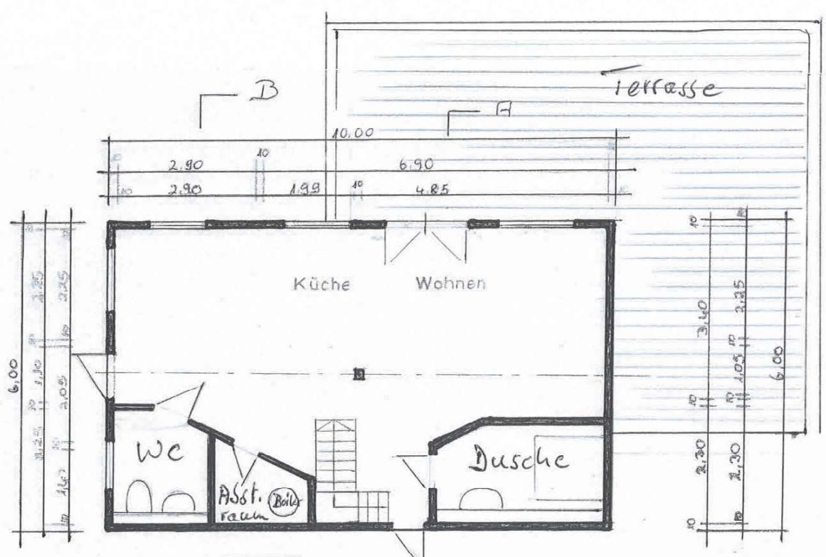
ERDGESCHOSS
