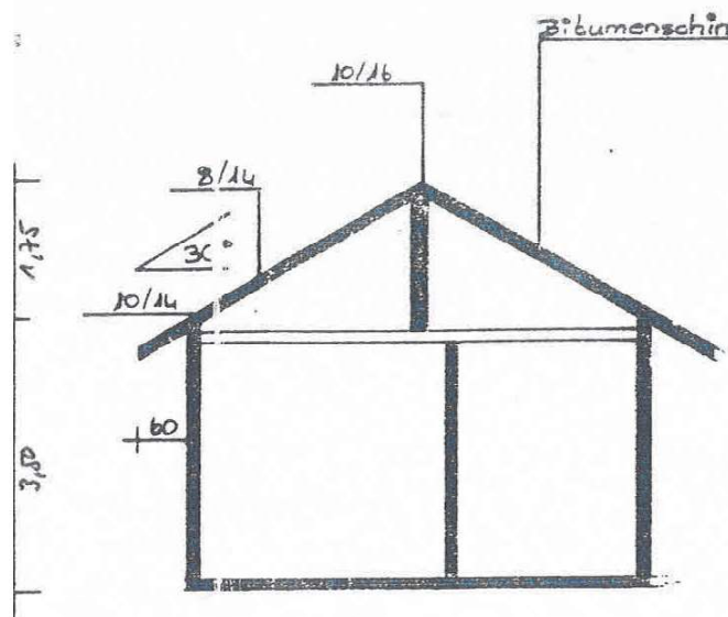
SCHNITT A-A
